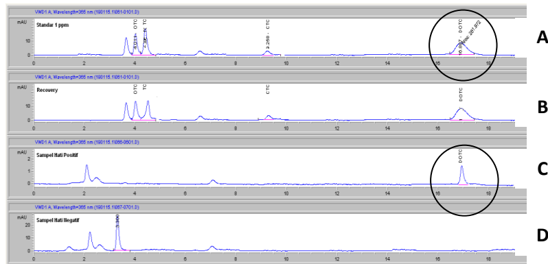
Gambar 2. Kromatogram sampel hati positif residu Doksisisiklin. Kromatogram A: Standar Oksitetrasiklin (OTC) RT 4.011; Standar Tetrasiklin (TC) RT 4.389; Standar Klortetrasiklin (CTC) RT 9.258; Standar Doksisisiklin (DOTC) RT 16.887; Kromatogram B: Recovery; Kromatogram C: Sampel hati positif mengandung residu Doksisisiklin pada RT 16.832; Kromatogram D: Sampel hati negatif mengandung residu golongan Tetrasiklin.
